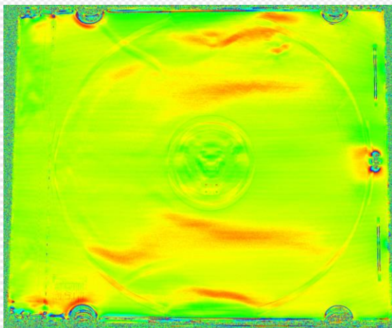
CD ケース ゆがみ分布
